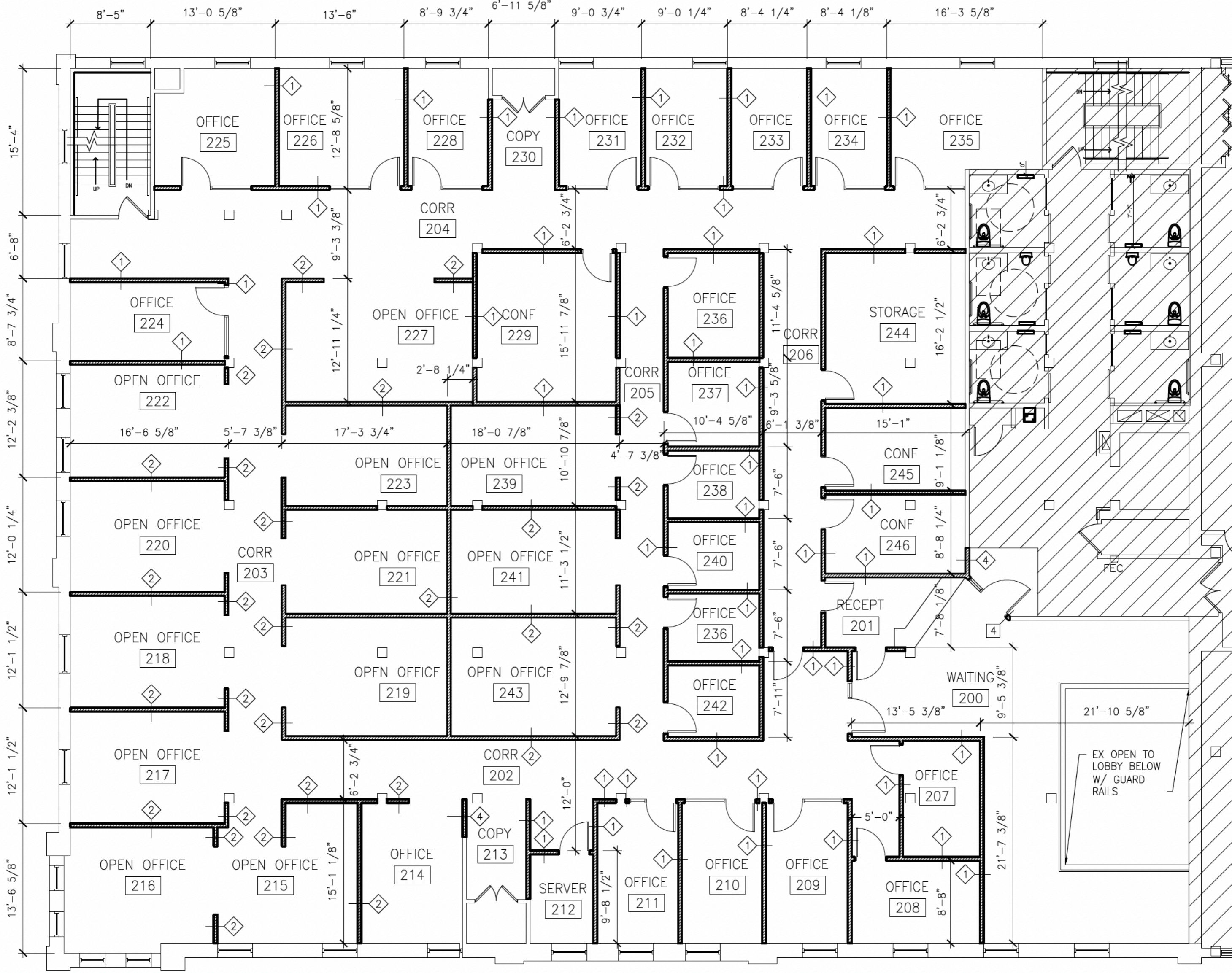
2 SECOND FL PLAN A-101 SCALE: 1/8" = 1'-0"
