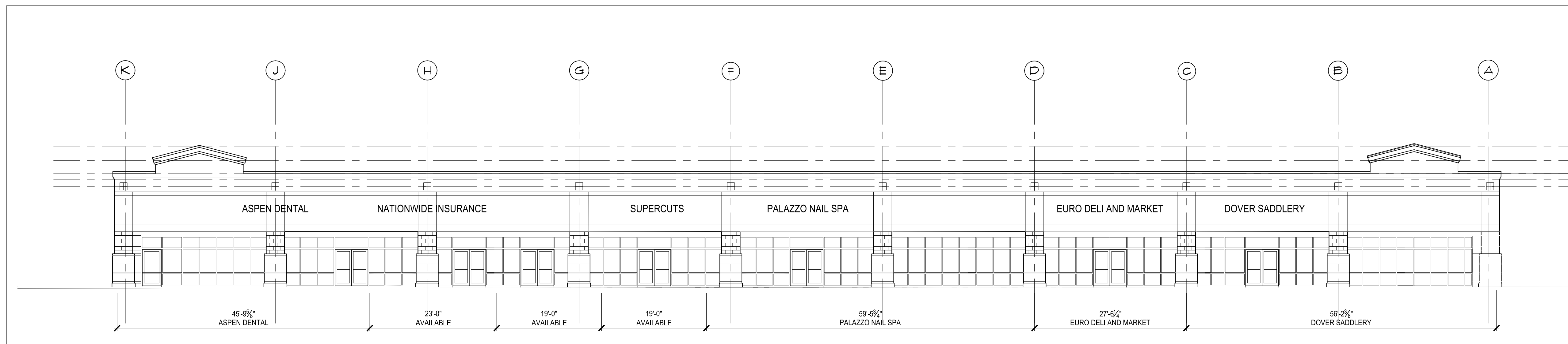
ELEVATION
