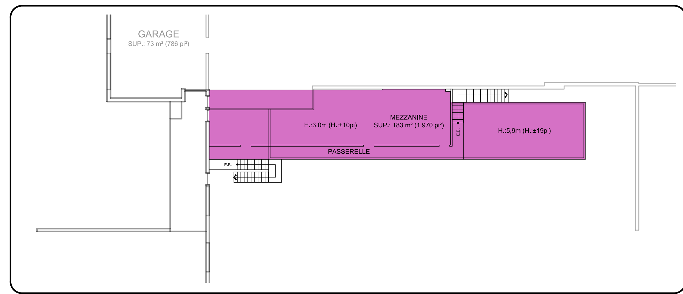
DÉTAIL - MEZZANINE
