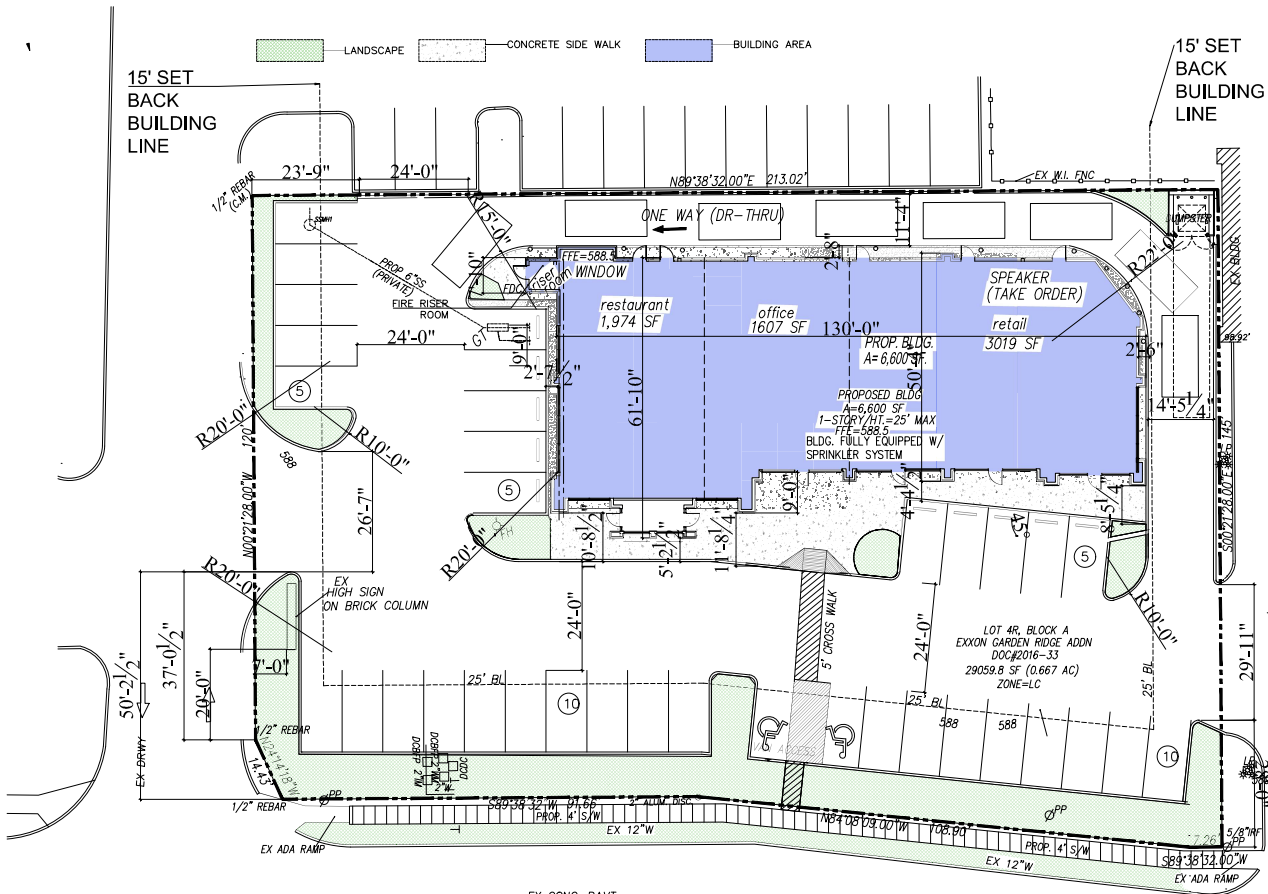
1 SITE PLAN 1"=10'
