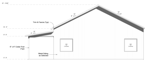
Right Elevation
