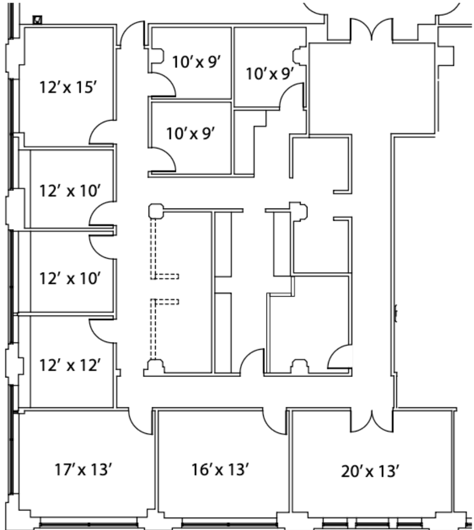
SUITE PLAN
