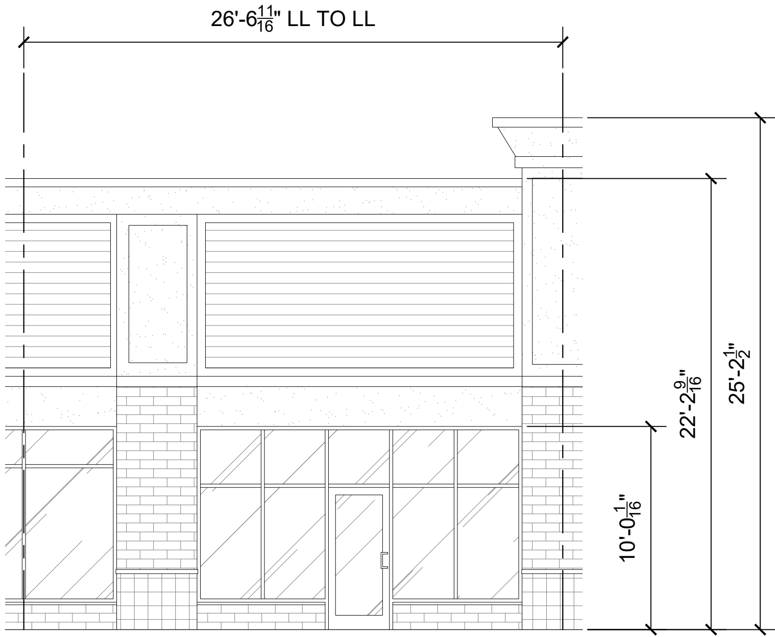
1 STOREFRONT ELEVATION A2 N.T.S.
