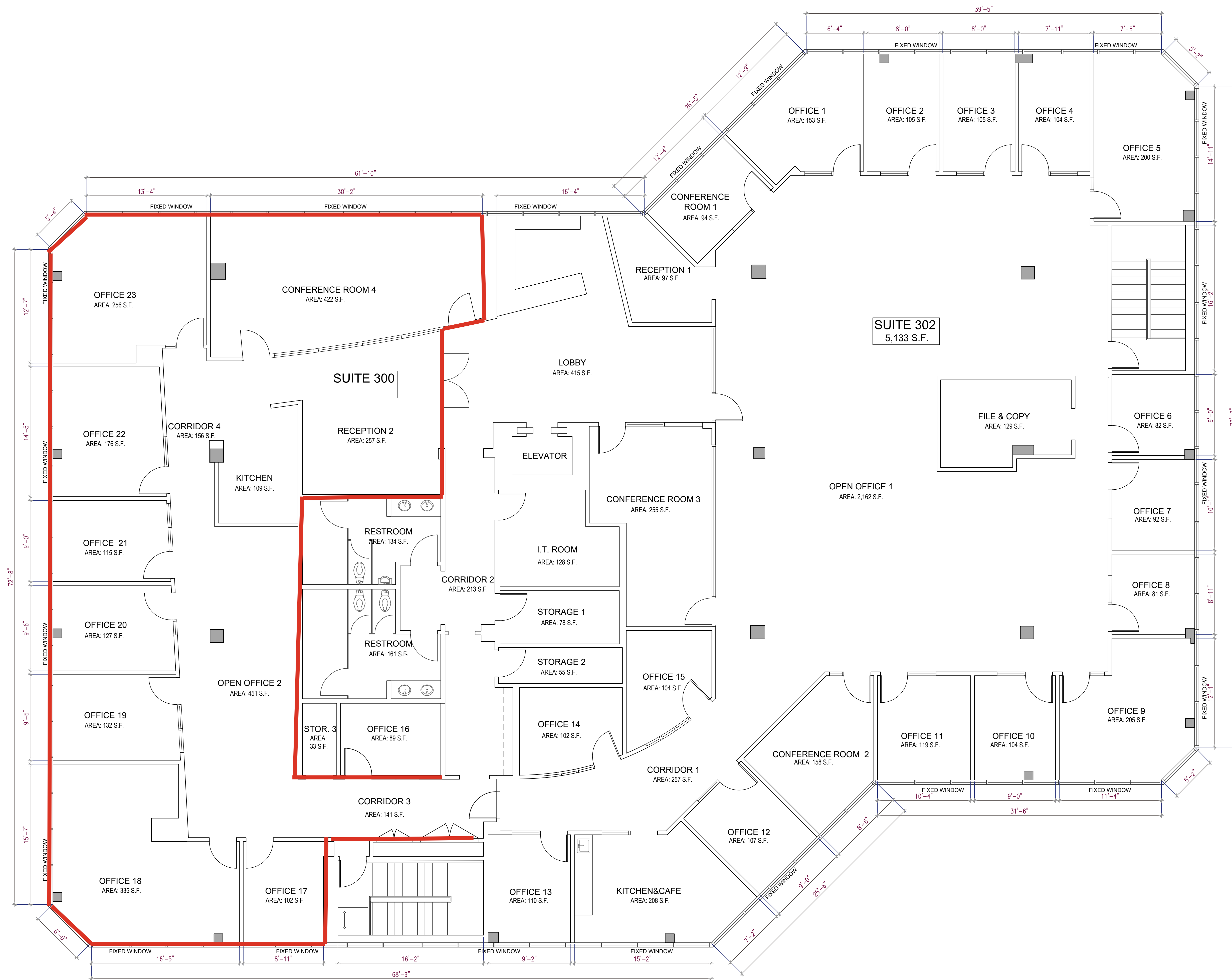
3RD FLOOR PLAN SCALE: N.T.S.
