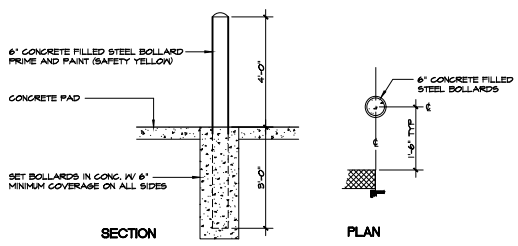
X BOLLARD DETAIL SCALE: 3/4" = 1'-0"
