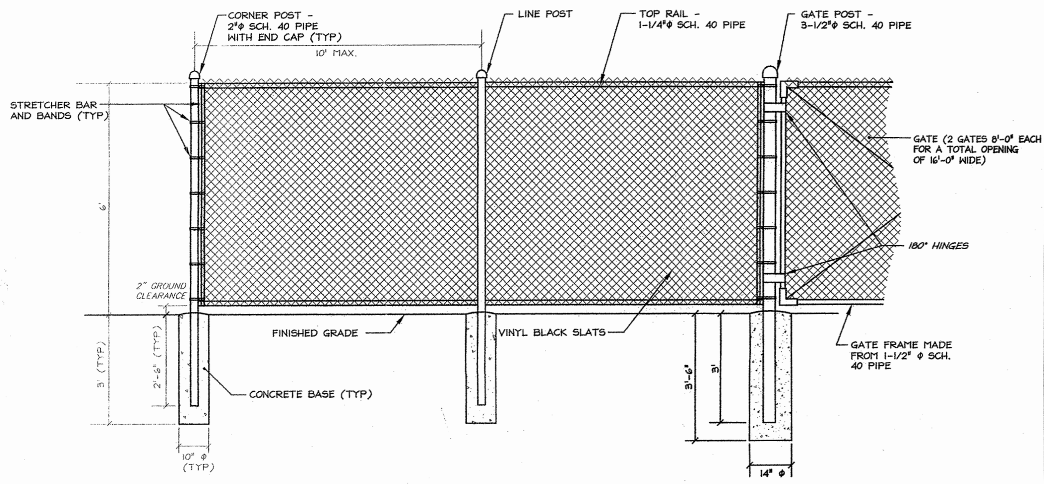
TRASH ENCLOSURE N.T.S.
