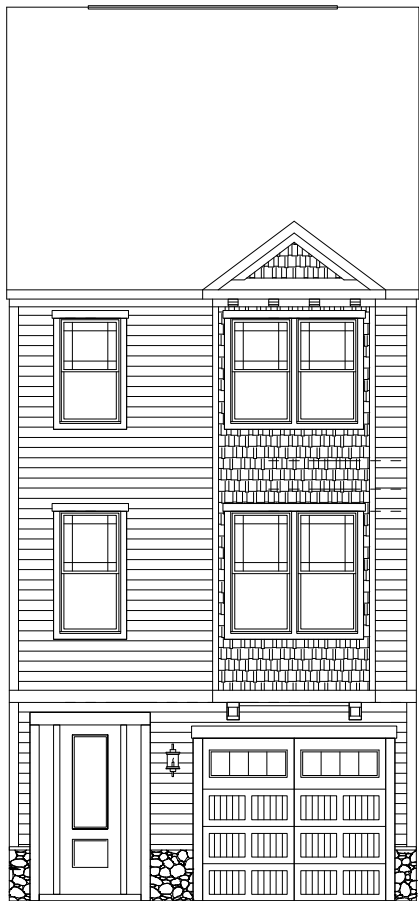
Elevation B
