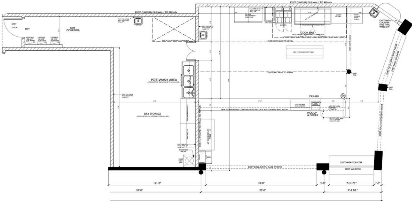
HAMBURGER SHOP 1,273 S.Q. FT.
