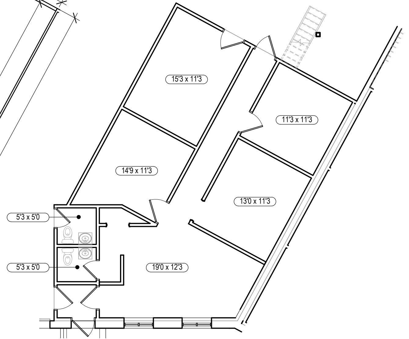
OFFICE PLAN Scale: 1/8" = 1'-0"
