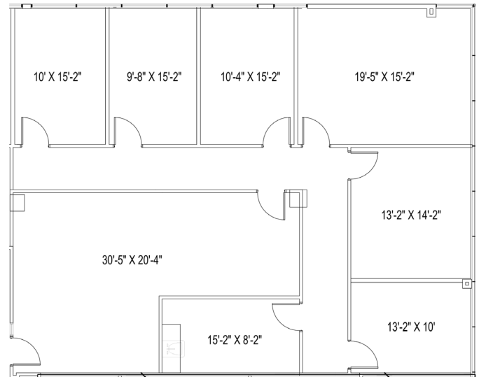
Suite 116 2,347 SF
