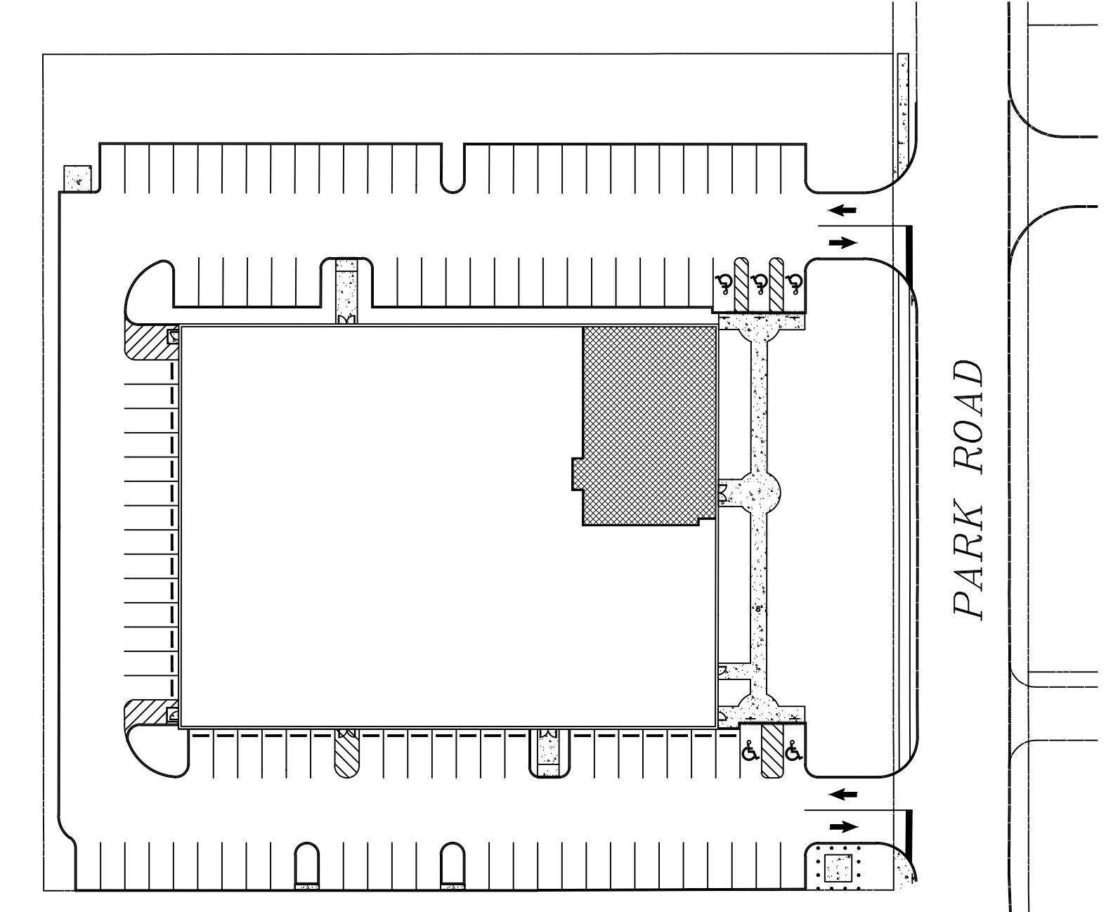
PLOT PLAN SCALE: 1" = 50'- 0"
