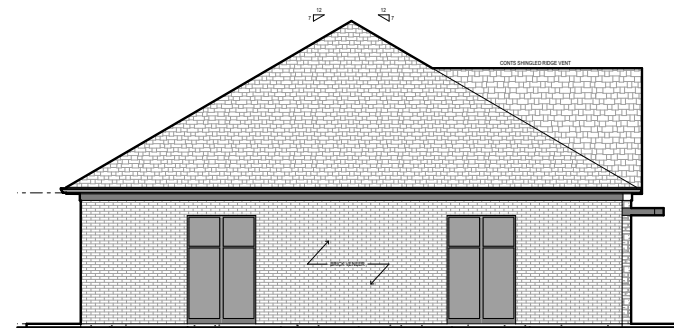
4 A-1 West Elevation SCALE: 3/16" = 1'-0"
